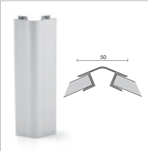
CODE giunzione 90°/135° rivestito 135 90°/135° covered end cap
