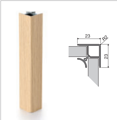
CODE giunzione 90° R2 157 90° R2 joint cap
