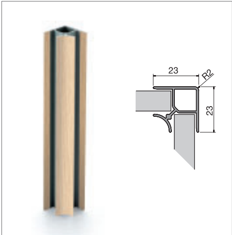
CODE giunzione 90° R2 doppio rivestimento 157 DR 90° R2 joint cap front and rear covering
