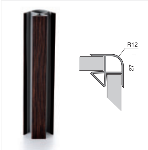
CODE giunzione 90° R12 doppio rivestimento 127 DR 90° R12 joint cap front and rear covering
