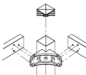
dettaglio del fissaggio delle travi alla gamba how to get beams fixed to legs
