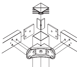
dettaglio del fissaggio delle travi alla gamba
