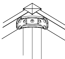
dettaglio del fissaggio delle travi alla gamba how to get beams fixed to legs
