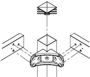
dettaglio del fissaggio delle travi alla gamba
