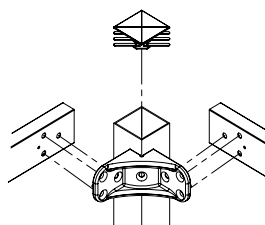
dettaglio del fissaggio delle travi alla gamba
