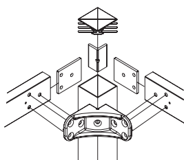
dettaglio del fissaggio delle travi alla gamba
